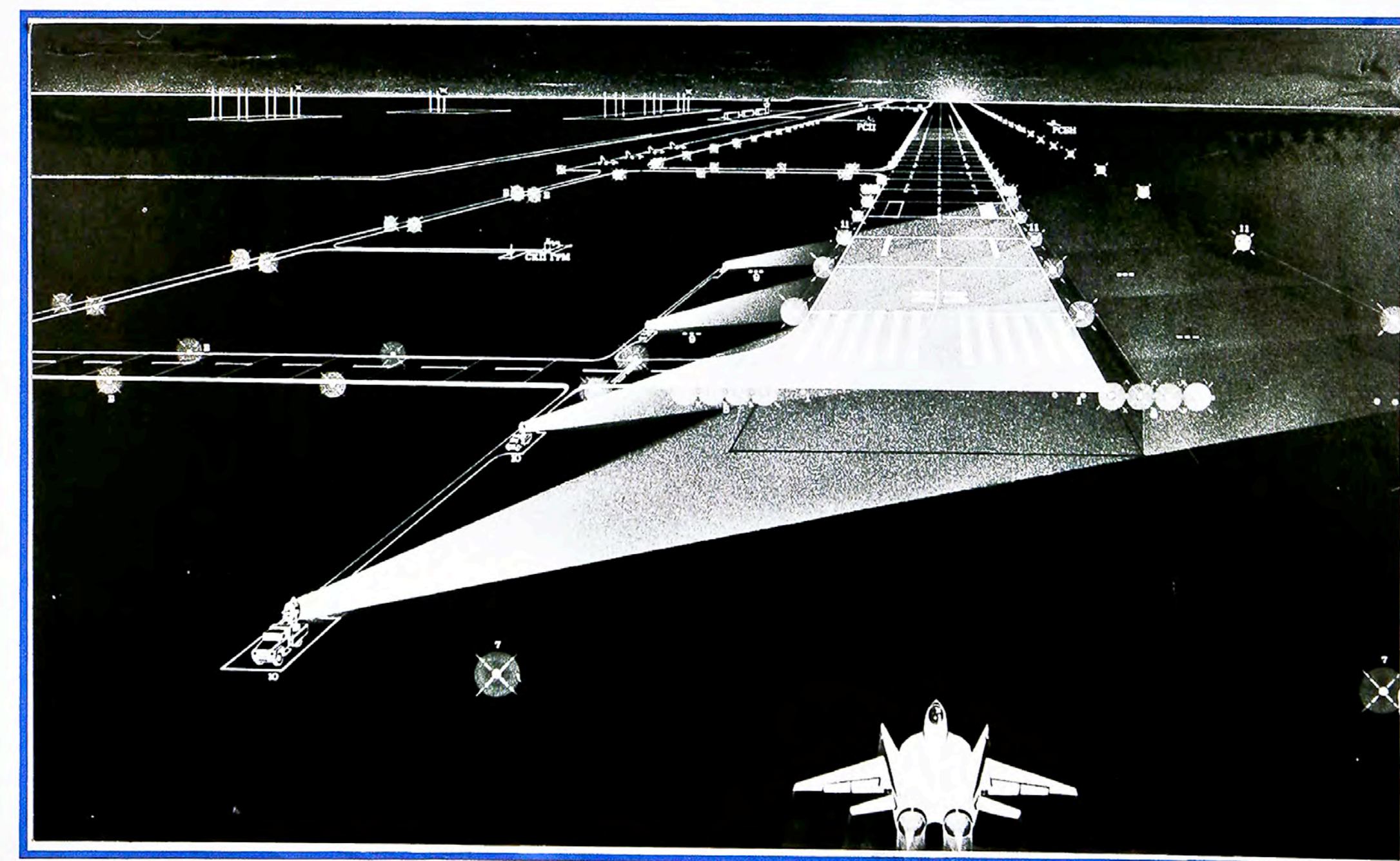
Світлотехнічне обладнання аеродрому типу "Свіча-3"
